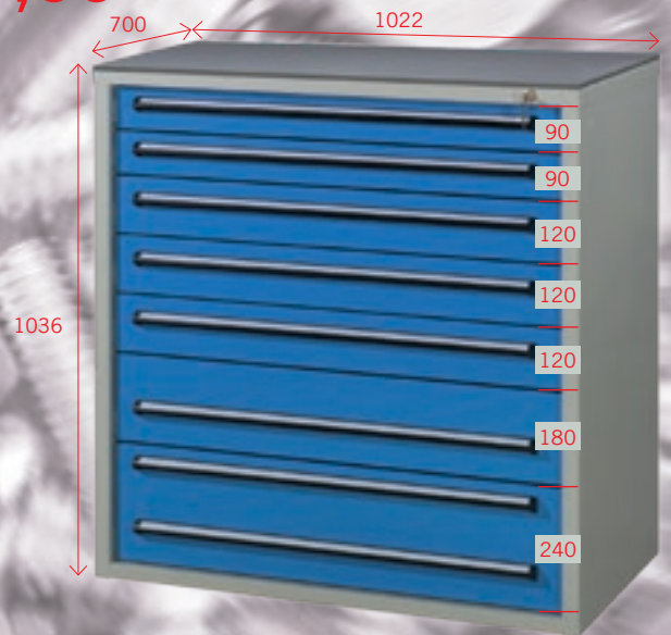
Schubladenschrank B7 1036/7
