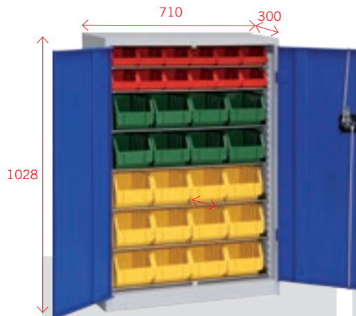
Regalschrank für Sichtlagerkästen Mod 1 HxB(mm) 1028x710x300
