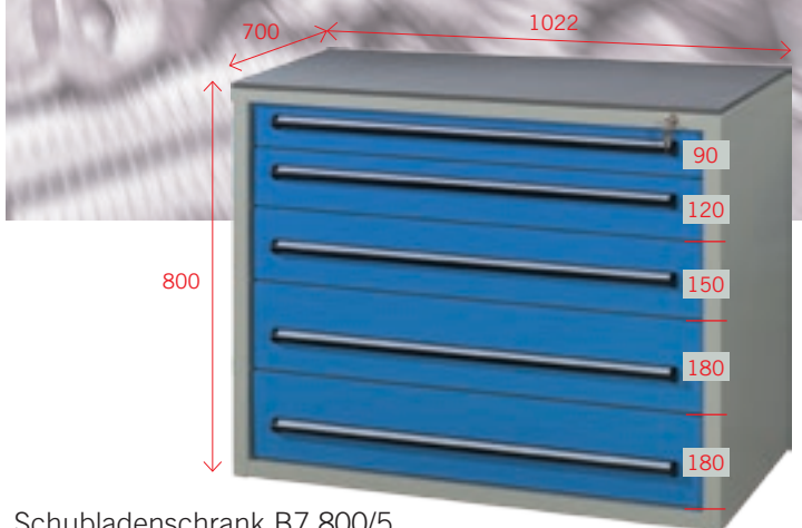
Schubladenschrank B7 800/5
