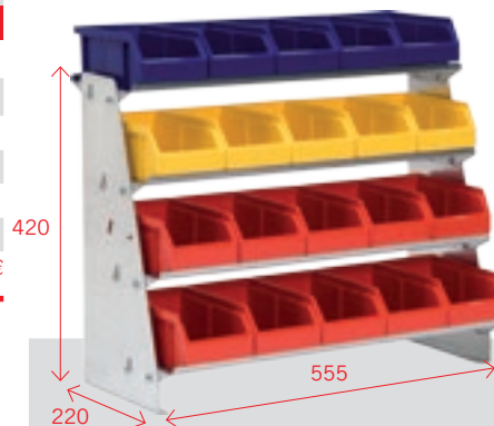
Tischständer für Sichtlagerkästen Mod 2 HxBxT(mm) 420x555x220
