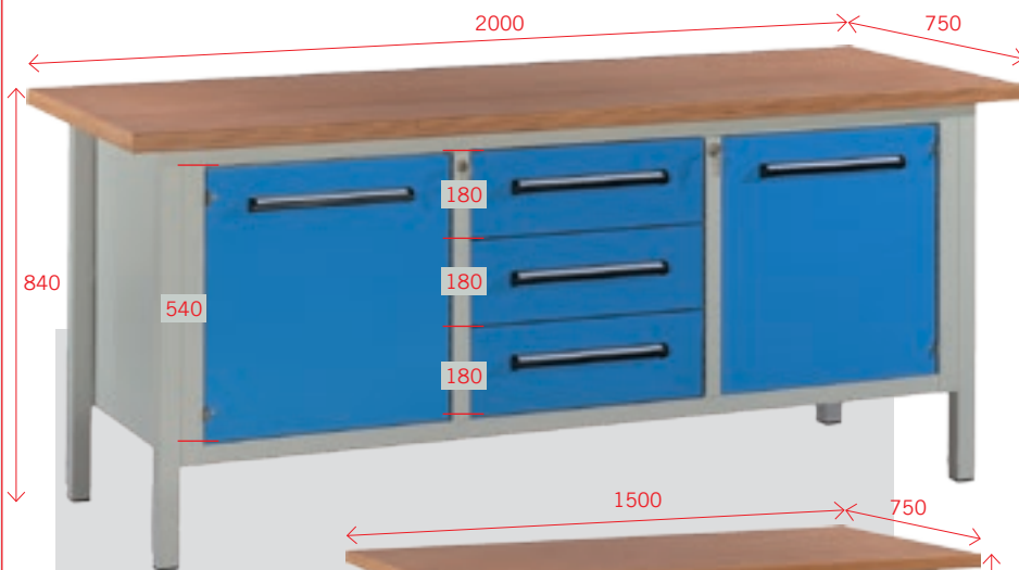
Kastenwerkbank 1500 2/3
