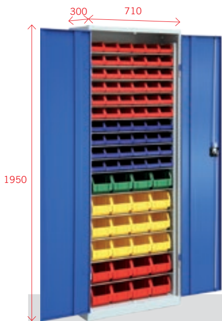
Regalschrank für Sichtlagerkästen Mod 3 HxBxT(mm) 1950x710x300
