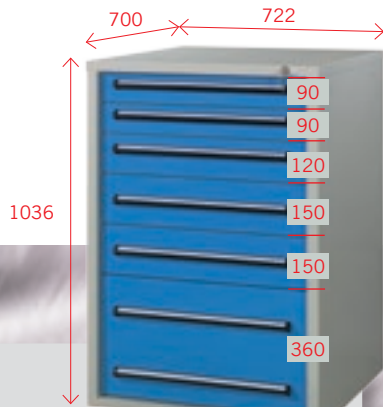
Schubladenschrank S7 1036/6 HxBxT(mm) 1036x722x700
